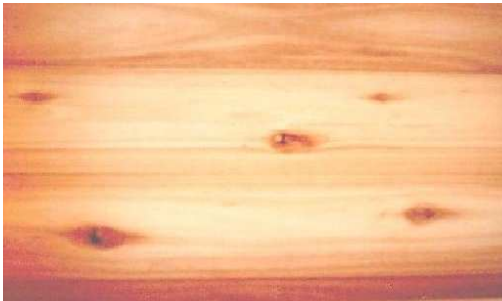
Figura 19 – Nós mortos associados com bolsas de resina, em tábuas de Eucalyptus grandis , na serraria da CAF Santa Bárbara Ltda, em Martinho Campos, MG.
